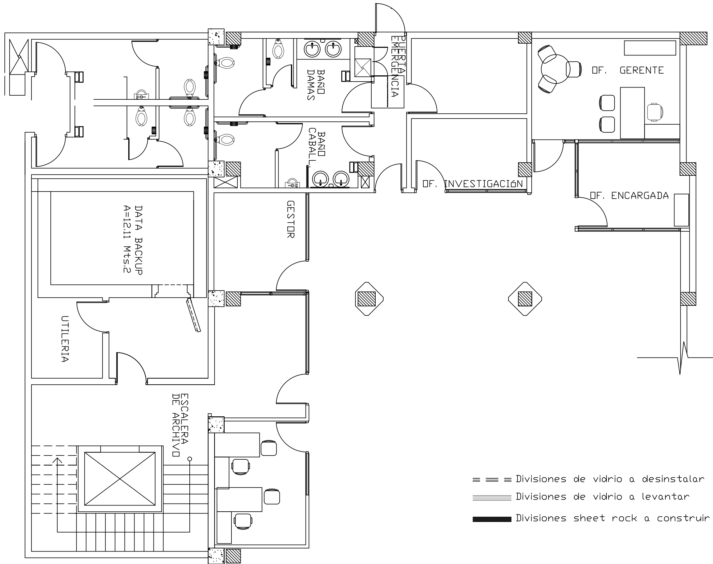
09 PLANTA AMUEBLADA AR- 09 REGISTRO INMOBILIARIO, 1ER. NIVEL SEDE CENTRAL
