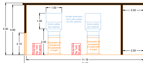
Sección 1-1'
