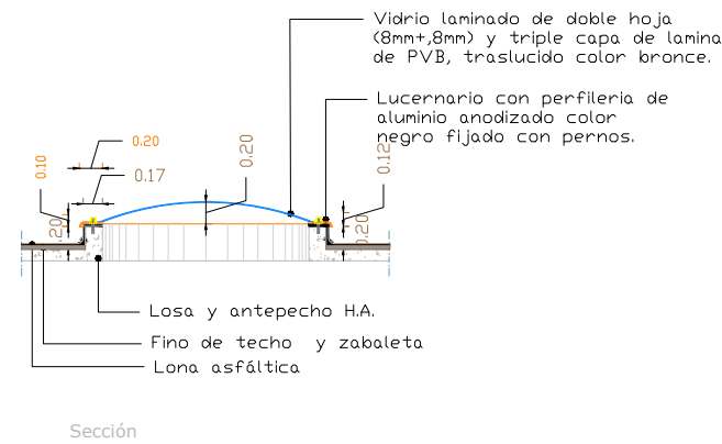
Sección
