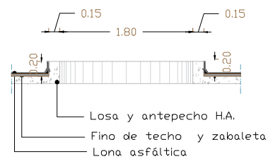
Sección tipo hueco de losa
