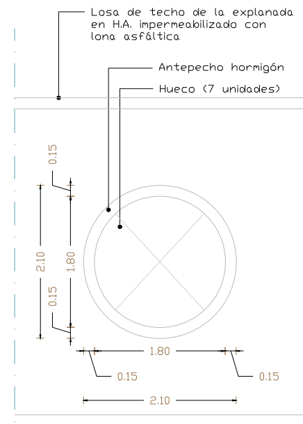
Planta tipo hueco de losa
